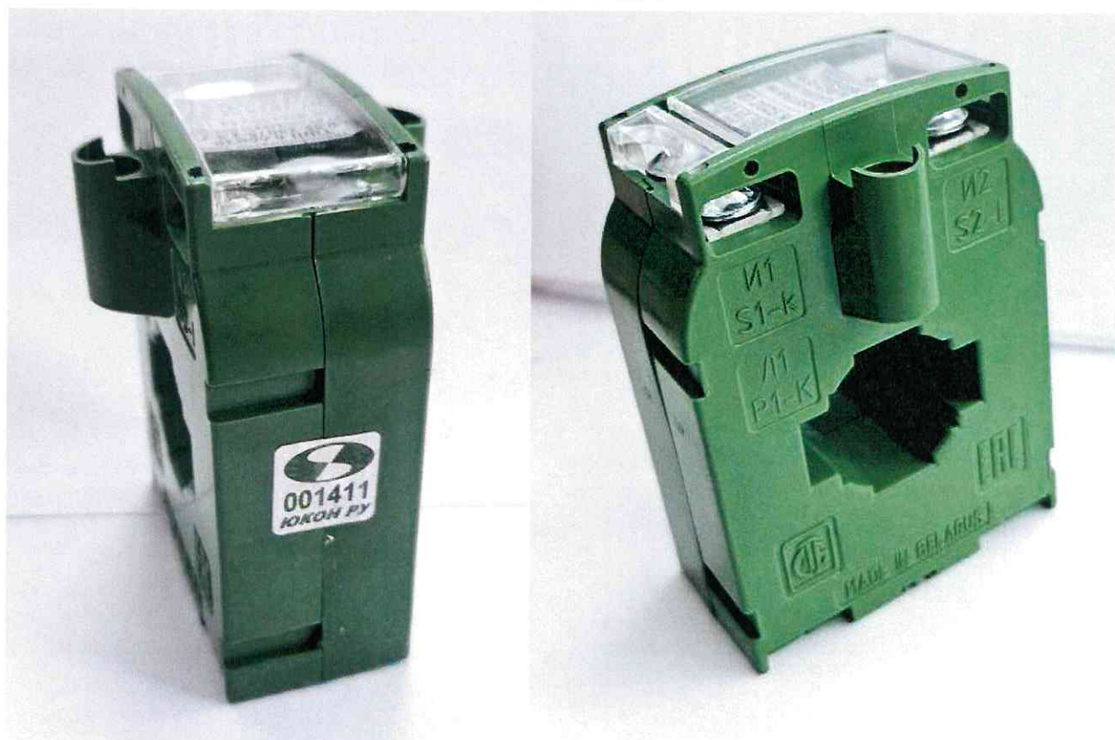
Рисунок 1.1 – Внешний вид трансформатора тока ТШП-0,66м30
