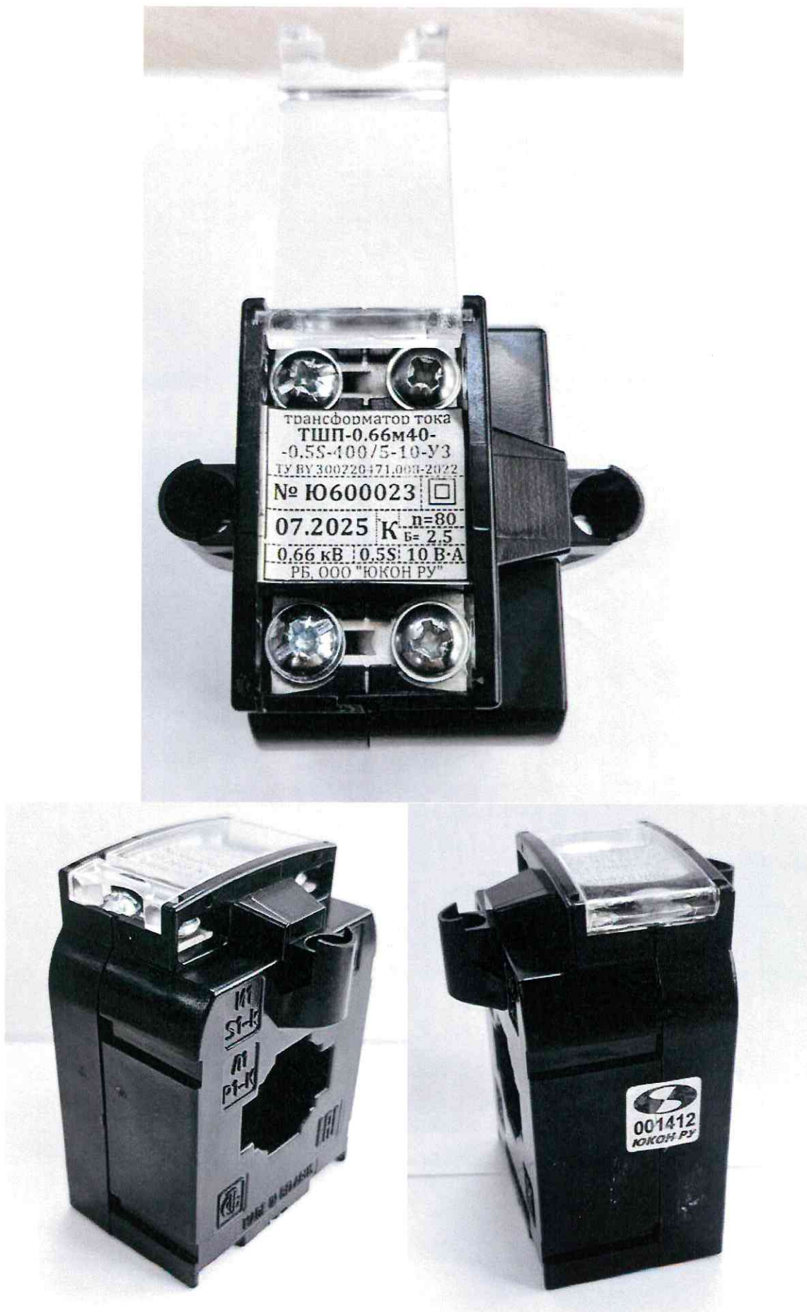
Рисунок 1.2 – Внешний вид трансформатора тока ТШП-0,66м40
